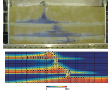
地盤中での非水溶性物質の浸透挙動評価
